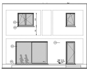
Achtergevel
