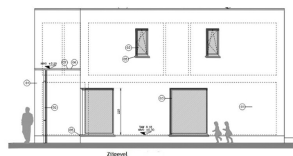
Zijgevel
